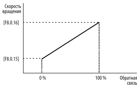
Рисунок 167 – соответствие скорости вращения электродвигателя значению сигнала обратной связи.
