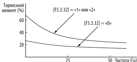
Рисунок 147 – изменение тормозного момента после применения торможения магнитным потоком.
