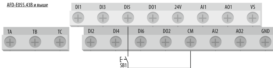
Рисунок 53 – схема подключения цепей управления при [F0.0.00] = «1» для AFD-E055.43B и выше.
