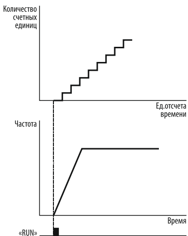
Рисунок 124 – запуск таймера при запуске электродвигателя.
