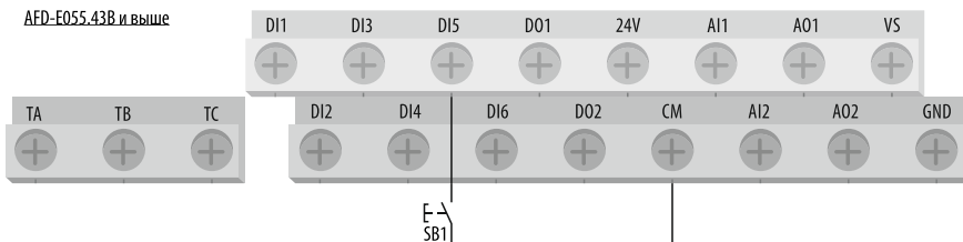
Рисунок 54 – схема подключения цепей управления при [F0.0.00] = «2» .
