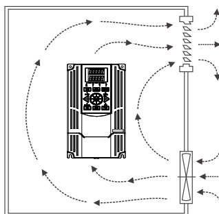
Рисунок 11 – расположение элементов системы дополнительной вентиляции.
